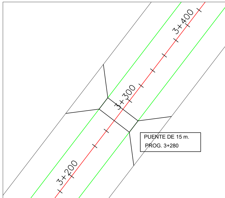
PLANTA DE UBICACIÓN
