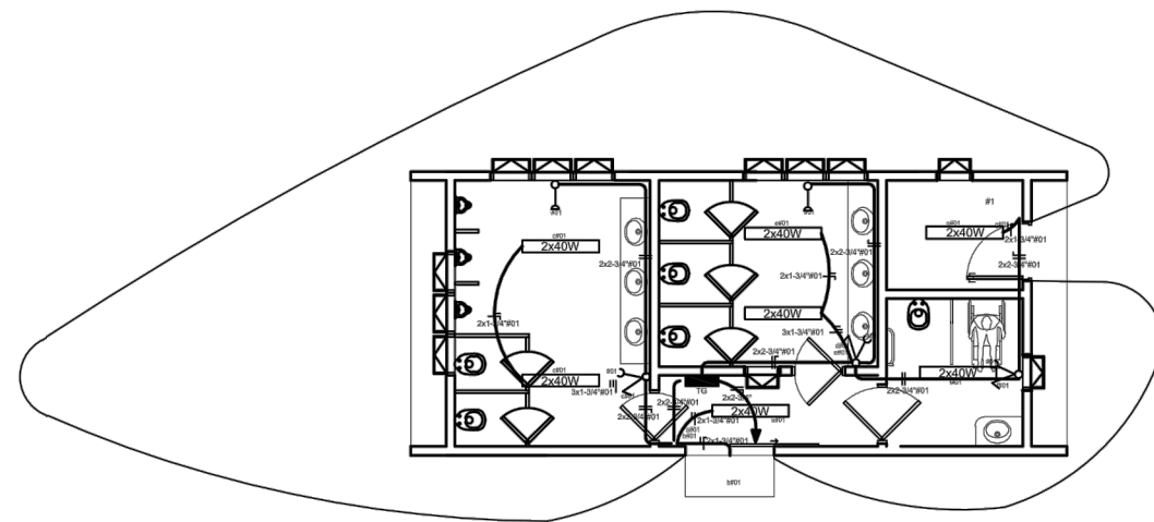
INSTALACIÓN ELÉCTRICA ESC. 1/75
